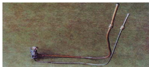
۵- نمایش مجموعه پیلوت (شمک - ترموکوپل)
